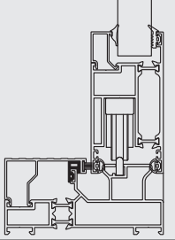
FTL30 - KAPAK DESTEK FİTİLİ / 74 gr FTL30 - ADAPTER GASKET / 74 gr
