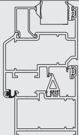
FTL05 - BİNİ FİTİLİ / 30 gr FTL05 - ACOUSTICAL GASKET INSIDE / 30 gr
