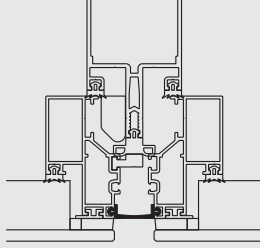
FTL25 - KULAK FİTİLİ / 44 gr FTL25 - SEALING GASKET / 44 gr
