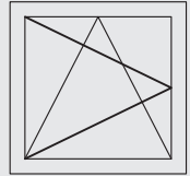
ÇİFT AÇILIM AKSESUARLARI 9 AKS-PVC KANALLI TILT AND TURN MECHANISM-FOR PVC ACC
