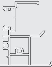
ADP02 - ALT ADAPTÖR KAPAĞI 55.A67.16 PROFİLİ İÇİN ADP02 - ADAPTER CAP BOTTOM FOR 55.A67.16
