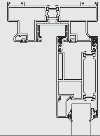
FTL28 - ÜST BİNİ FİTİLİ / 31 gr FTL28 - ACOUSTICAL GASKET / 31 gr
