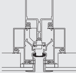
FTL24 - KULAK FİTİLİ / 38 gr FTL24 - SEALING GASKET / 38 gr
