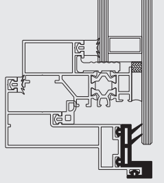
FTL36 - BİNİ FİTİLİ / 326 gr FTL36 - ACOUSTICAL GASKET / 326 gr
