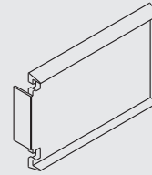
ENJ02.080 - 80'LİK ENJEKSİYON BAĞLANTI ENJ02.080 - TRANSOM CONNECTION PART (80 mm)
