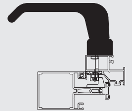
KOL04 - BÜKÜMLÜ CEPHE KOLU - YERLİ KOL04 - HANDLE
