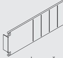
ENJ01 - ENJEKSİYON BAĞLANTI ENJ01 - TRANSOM CONNECTION PART
