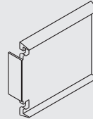
ENJ02.060 - 60'LİK ENJEKSİYON BAĞLANTI ENJ02.060 - TRANSOM CONNECTION PART (60 mm)
