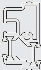
ADP06 - ALT ADAPTÖR KAPAĞI ST113.A01.18 PROFİLİ İÇİN ADP06 - ADAPTER CAP BOTTOM FOR ST113.A01.18
