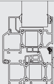
FTL06 - BİNİ FİTİLİ / 30 gr FTL06 - ACOUSTICAL GASKET INSIDE / 30 gr
