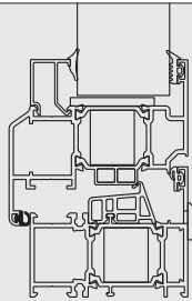
FTL05 - BİNİ FİTİLİ / 30 gr FTL05 - ACOUSTICAL GASKET INSIDE / 30 gr
