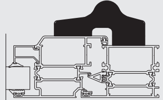
HNG03 - KAPI MENTEŞESİ HNG03 - DOOR HINGE
