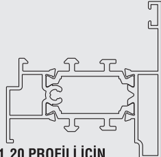
ADP10 - ALT ADAPTÖR KAPAĞI PT55.A61.20 PROFİLİ İÇİN ADP10 - ADAPTER CAP BOTTOM FOR PT55.A61.20
