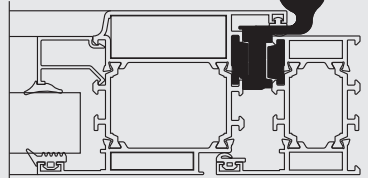
HNG02 - KAPI MENTEŞESİ HNG02 - DOOR HINGE
